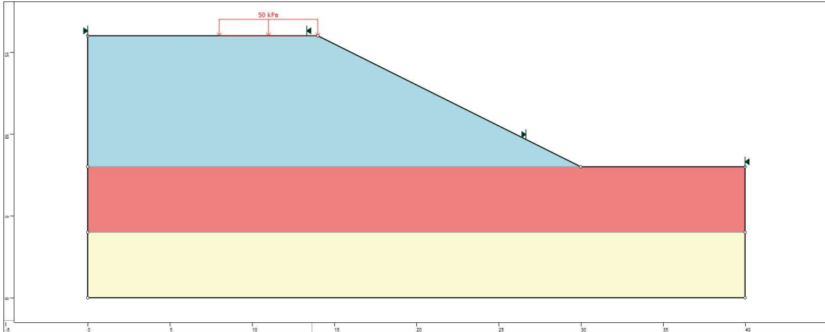
Рисунок 6- Вид модели с приложенной нагрузкой.
